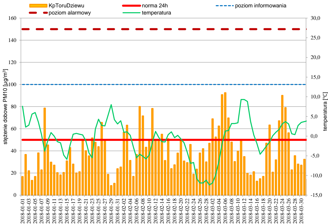
Rysunek 13. Porównanie przebiegu zmienności stężeń 24-godz. PM10 w I kwartale 2018 r. w Toruniu z temperaturą 52
