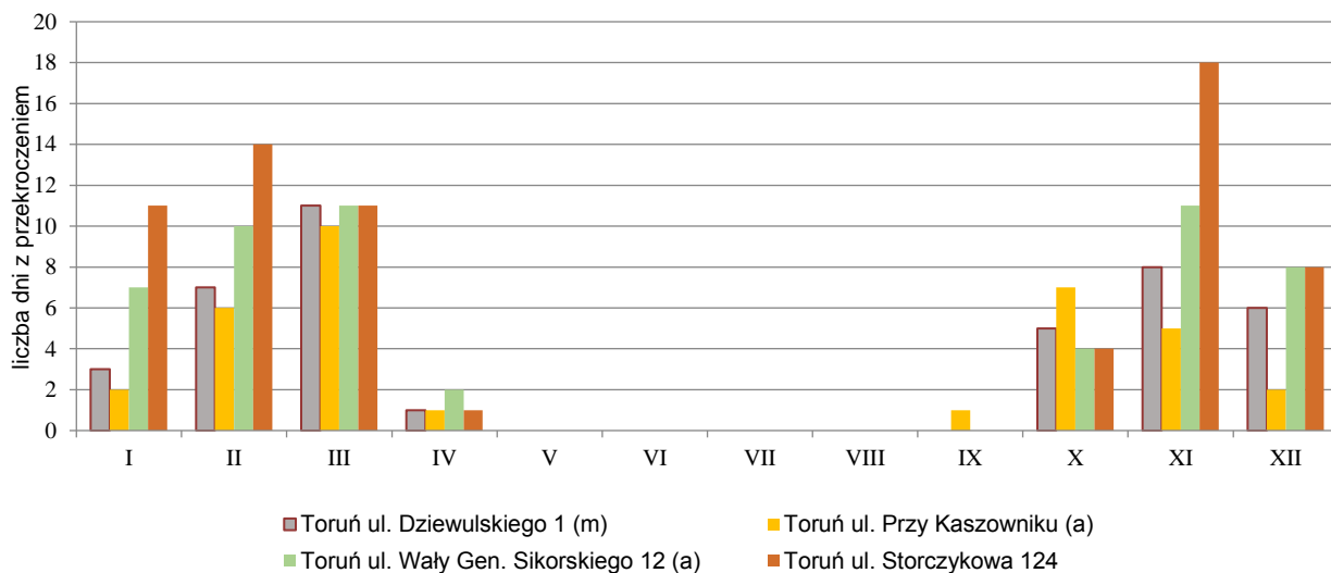
Rysunek 6. Liczba dni z przekroczeniem dopuszczalnego stężenia 24-godz. PM10 w 2018 r. 42
