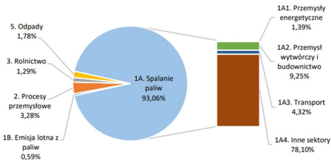
Rysunek 4. Udziały poszczególnych rodzajów emitentów w emisji pyłu zawieszono PM 2,5 w 2020 r. 37
