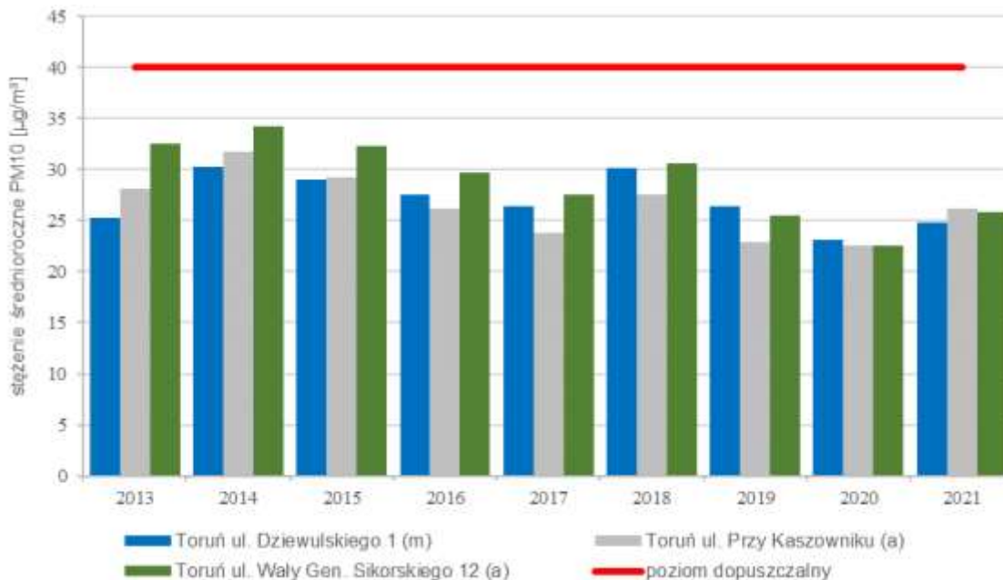
Rysunek 8. Stężenie średnioroczne PM10 w strefie miasto Toruń 44
