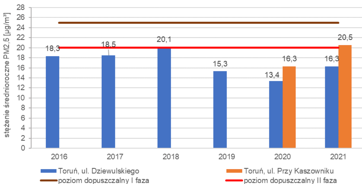
Rysunek 16. Stężenia średnioroczne pyłu zawieszonego PM 2,5 w latach 2016-2021 w strefie miasto Toruń 55
