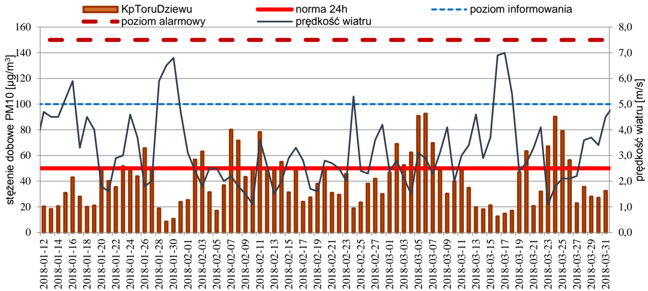
Rysunek 9. Porównanie przebiegu zmienności stężeń 24-godz. PM10 w I kwartale 2018 r. w Toruniu z prędkością wiatru 48
