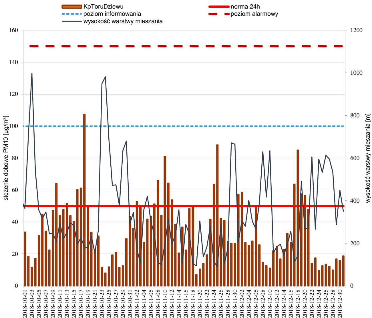
Rysunek 12. Porównanie przebiegu zmienności stężeń 24-godz. PM10 w IV kwartale 2018 r. w Toruniu z wysokością warstwy mieszanania 51
