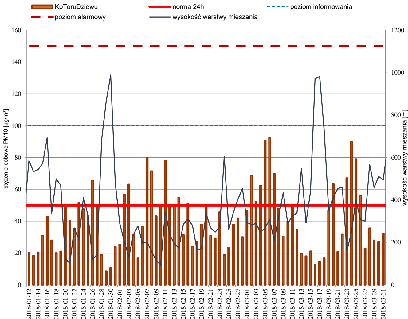
Rysunek 11. Porównanie przebiegu zmienności stężeń 24-godz. PM10 w I kwartale 2018 r. w Toruniu z wysokością warstwy mieszania 50
