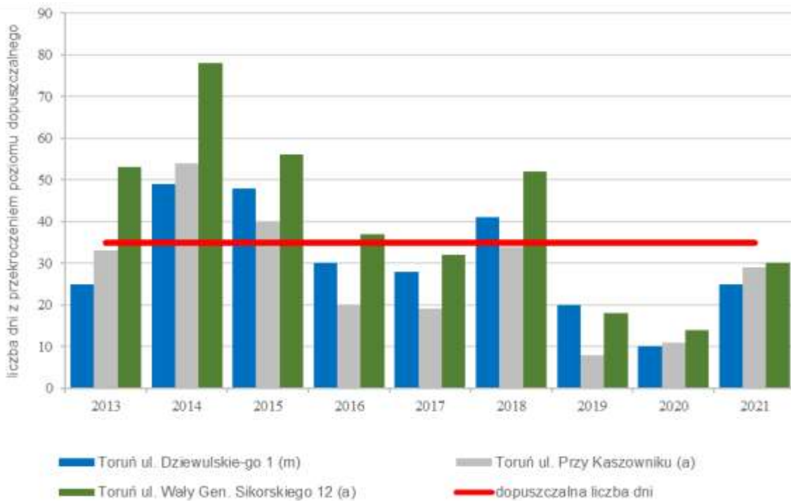
Rysunek 7. Liczba dni z przekroczeniem dopuszczalnego stężenia 24-godz. PM10 w strefie miasto Toruń w latach 2013-2021 43
