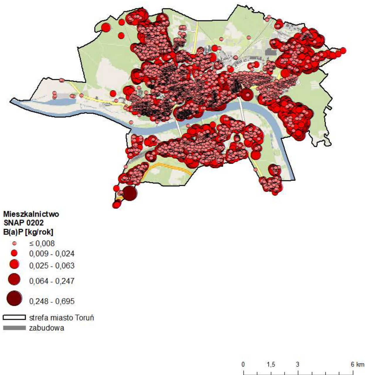
Rysunek 54. Emisja benzo(a)pirenu z mieszkalnictwa (SNAP 0202) w 2021 r. 134
