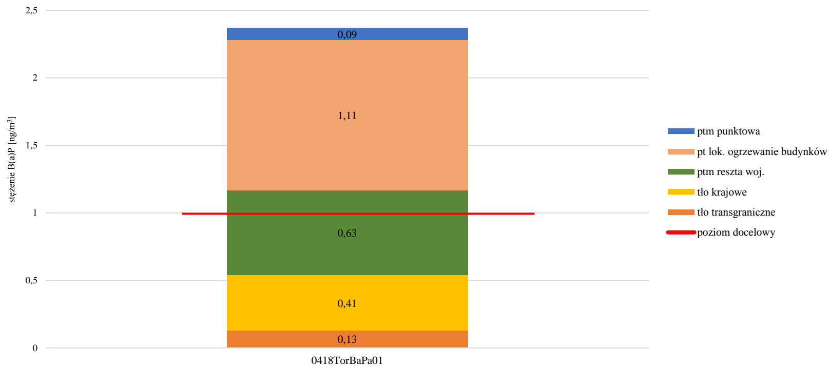
Rysunek 24. Obszar przekroczeń poziomu docelowego benzo(a)pirenu w Toruniu 77
