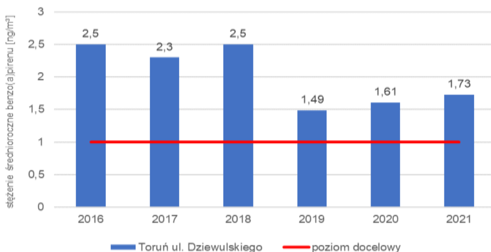
Rysunek 15. Stężenie średnioroczne benzo(a)pirenu w latach 2016-2021 w strefie miasto Toruń 54
