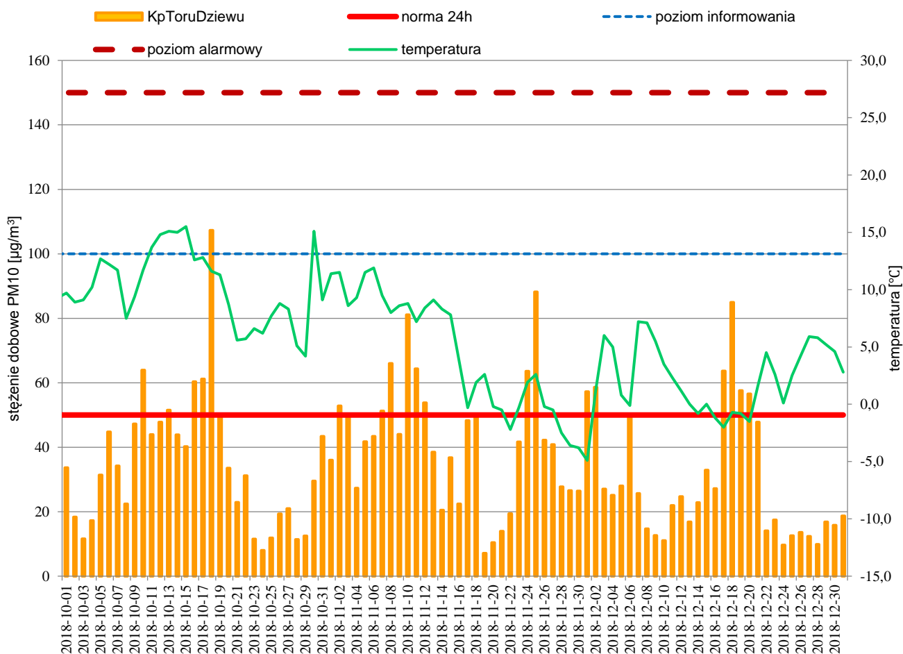
Rysunek 14. Porównanie przebiegu zmienności stężeń 24-godz. PM10 w IV kwartale 2018 r. w Toruniu z temperaturą 53
