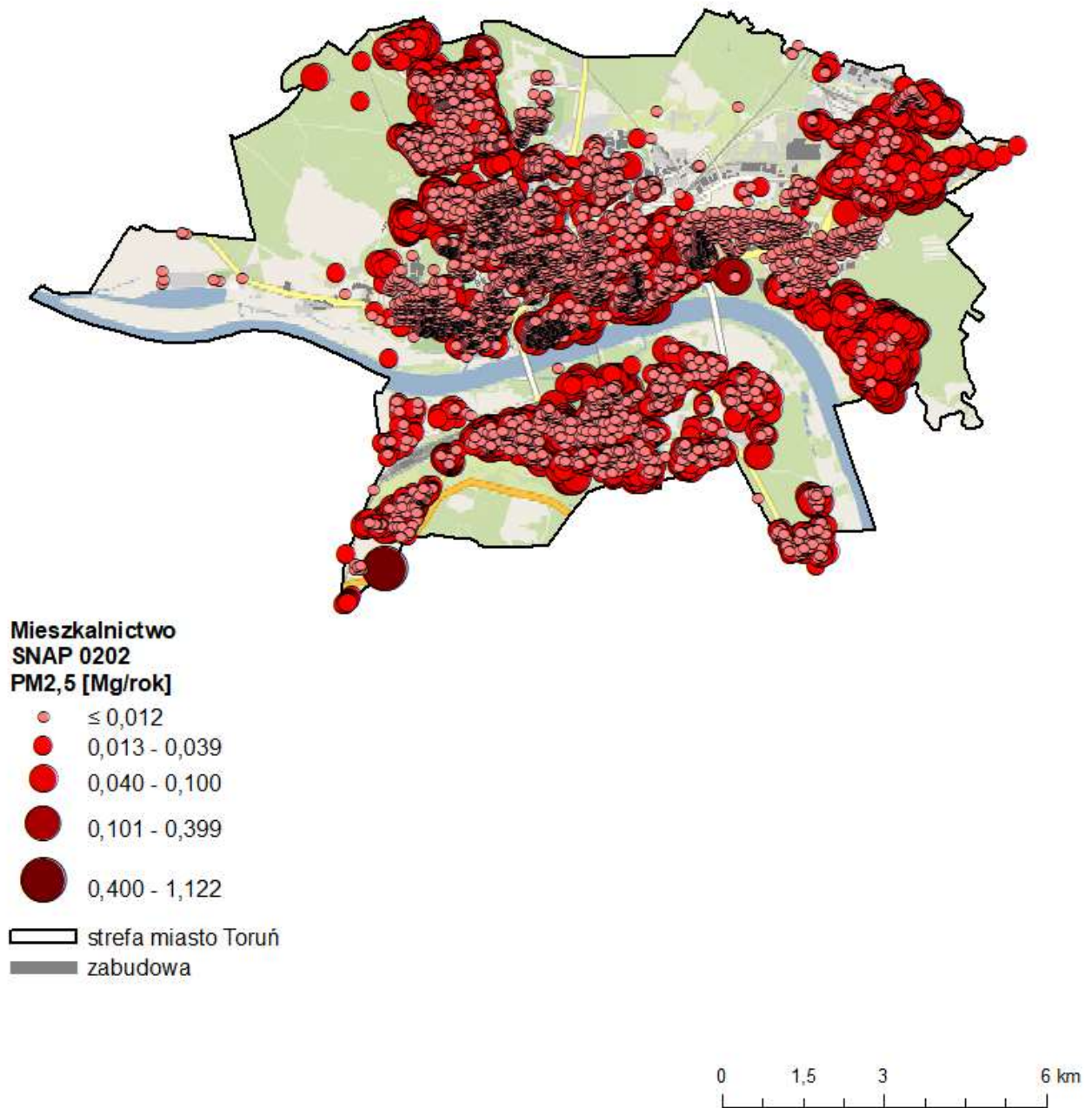
Rysunek 55. Emisja pyłu zawieszonego PM2,5 z mieszkalnictwa (SNAP 0202) w 2021 r. 135
