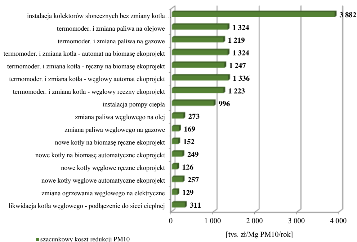
Rysunek 56. Porównanie szacunkowych, średnich wskaźników kosztów redukcji pyłu zawieszonego PM10 z indywidualnych systemów grzewczych 158
