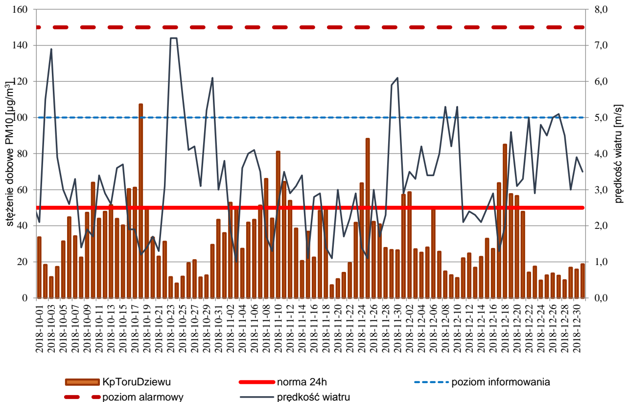
Rysunek 10. Porównanie przebiegu zmienności stężeń 24-godz. PM10 w IV kwartale 2018 r. w Toruniu z prędkością wiatru 49
