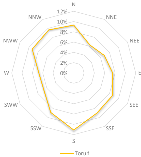
Rysunek 2. Róża wiatrów dla miasta Toruń w 2018 r. 28
